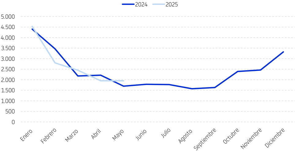
EVOLUCIÓN DISOLUCIONES
