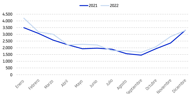
EVOLUCIÓN DISOLUCIONES
